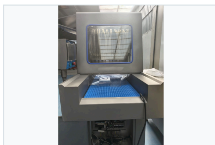
Esteira de saída e cabeçote
